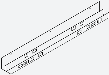
Calha
